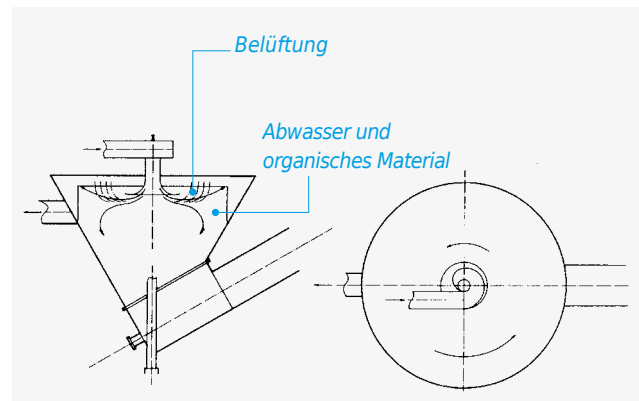
Prinzipskizze HUBER Coanda Sandklassierer RoSF3.
